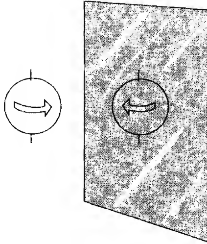
شكل خ-٤: تماثل الانعكاس: دوران الكرة في عالم المرآة هو نفسه مثل انعكاس الزمان لدورانها في العالم الواقعي.
